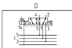
D = 5/2, monostabile con scheda bistabile
