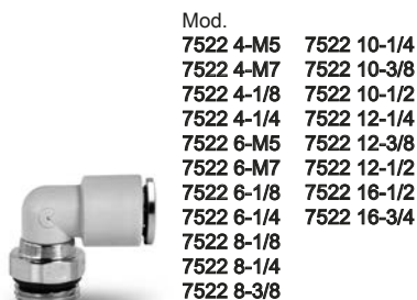
Gomito Girevole Metrico-Cilindrico Maschio
